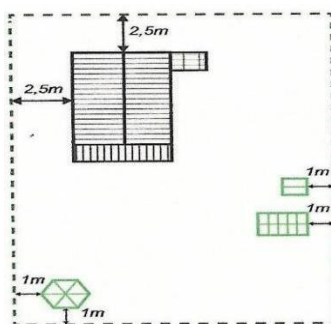
Indretning af havelod hvor skur er sammenbygget med kolonihavehus.
