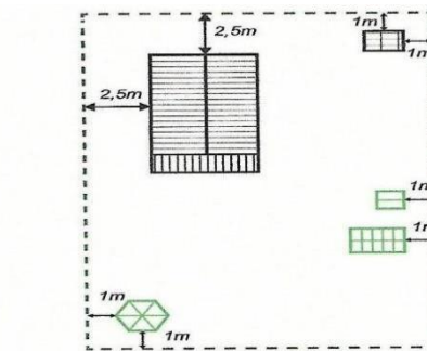
Indretning af havelod hvor skur er fritliggende.
